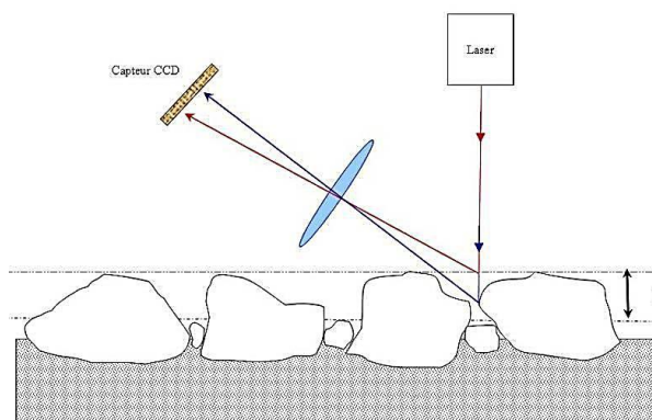
Principe de mesure de la macrotexture (PMP)
